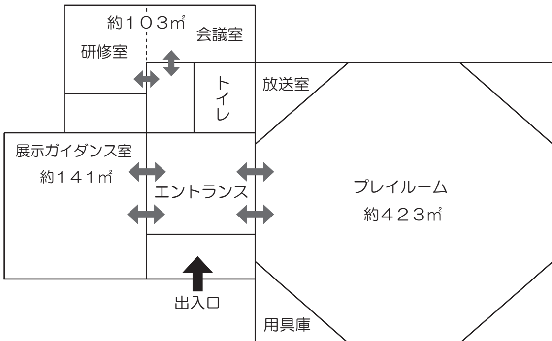
(2) 集会棟平面図
